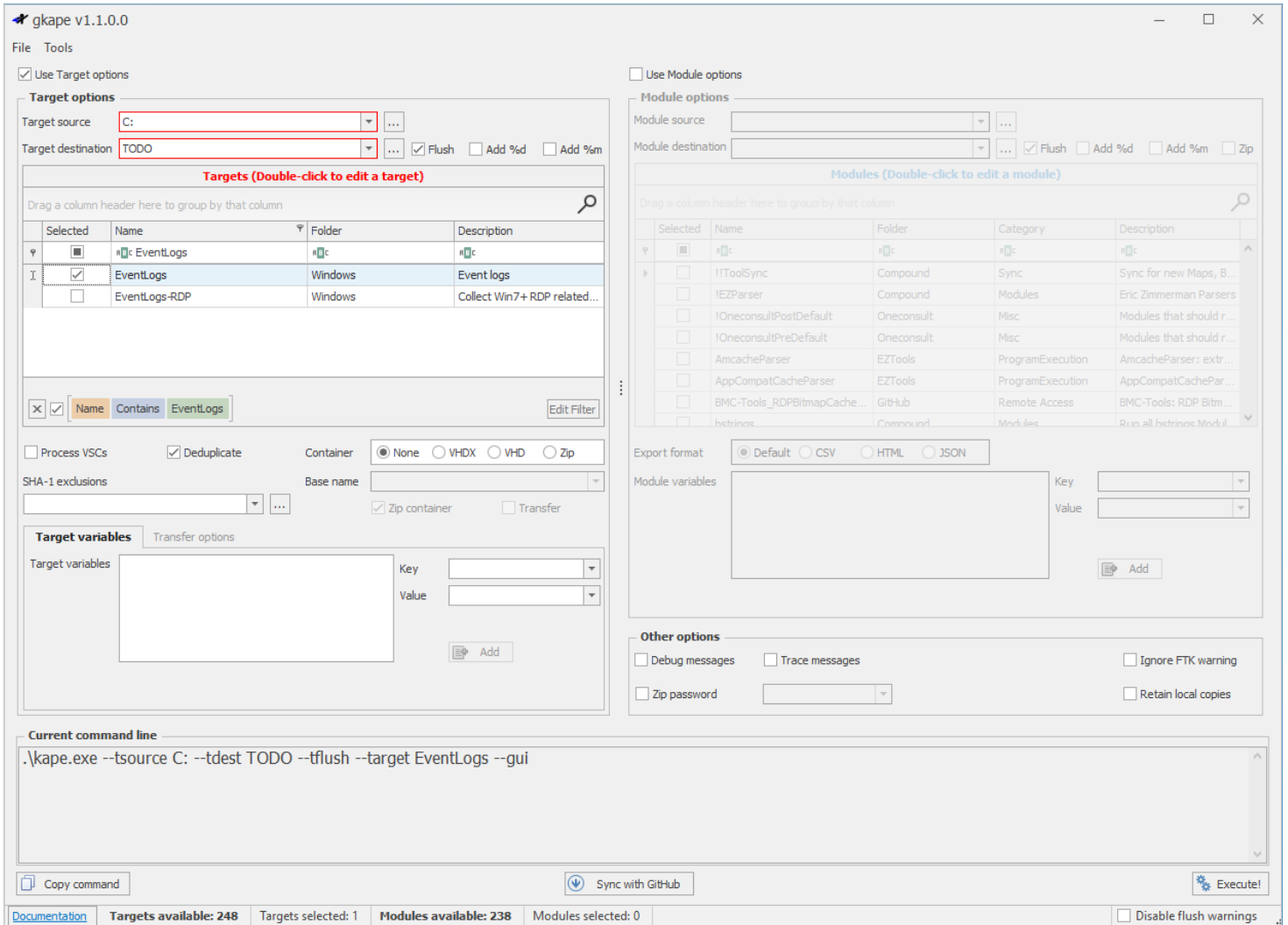
Beispielkonfiguration für das Sammeln der Windows-Ereignisprotokolle (Abb. 1)
